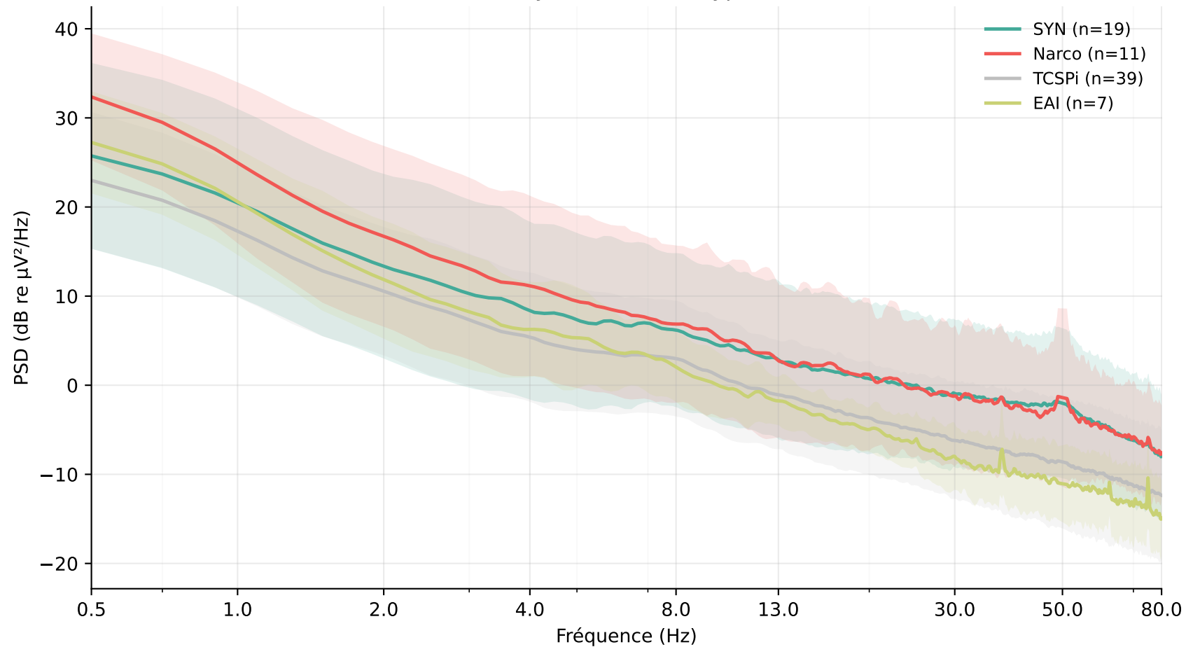
PSD moyen par groupe - T3-A1 (moyenne \pm écart-type)
