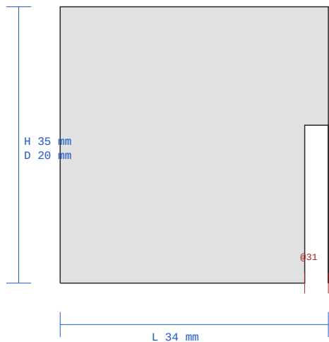
wv-5 x2 (depth-run) T 3 mm
