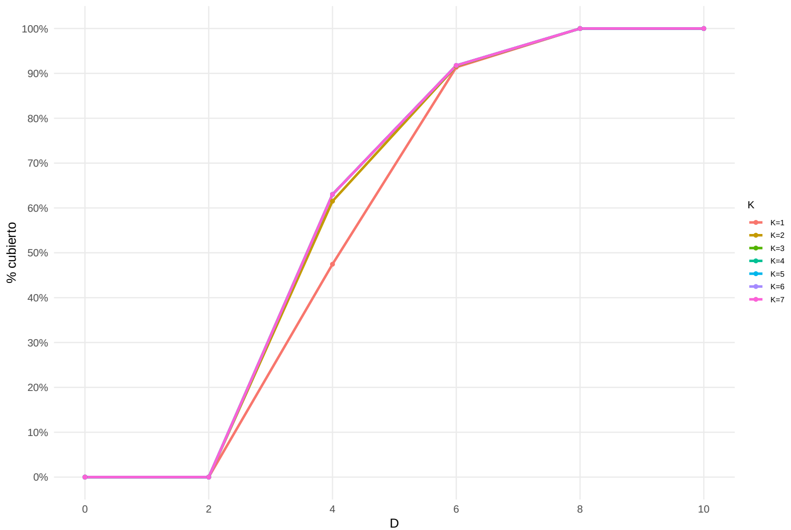
sins - ext - 10^{-9} (orden D=4)
