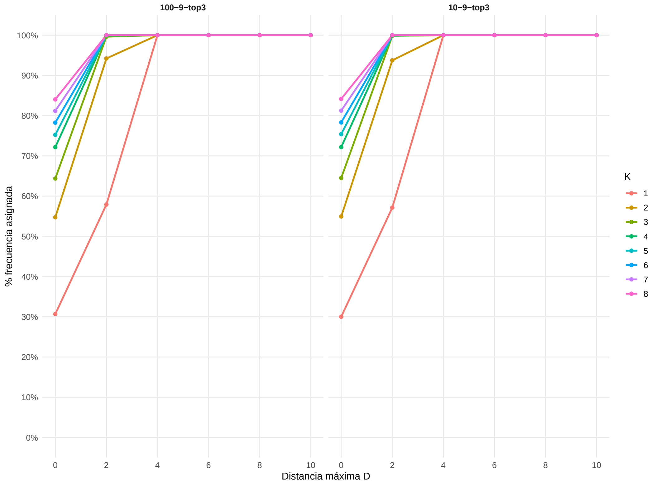
Greedy(3): % frecuencia asignada vs D para distintos K – EXT
