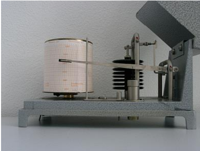
DWD marine barograph (photo Deutscher Wetterdienst)
