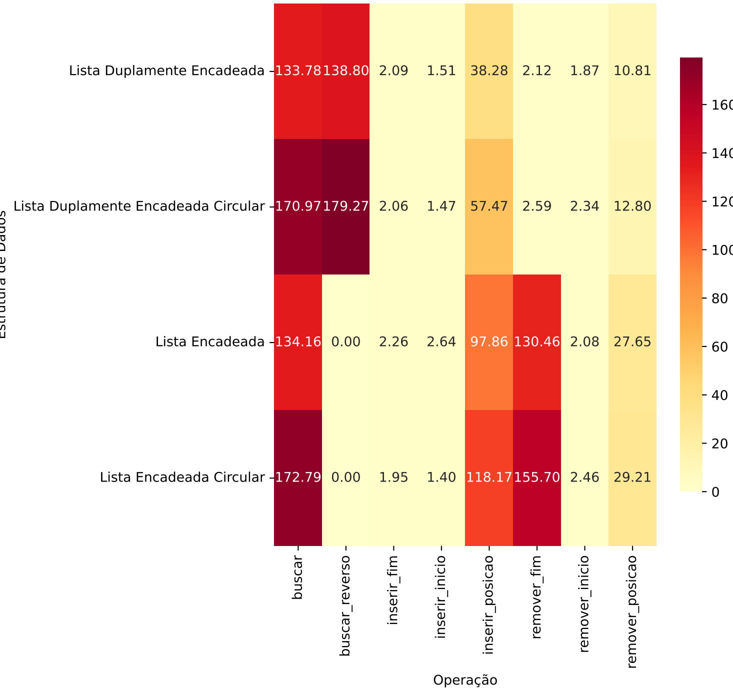
Linux - Tempo Total (ms)
