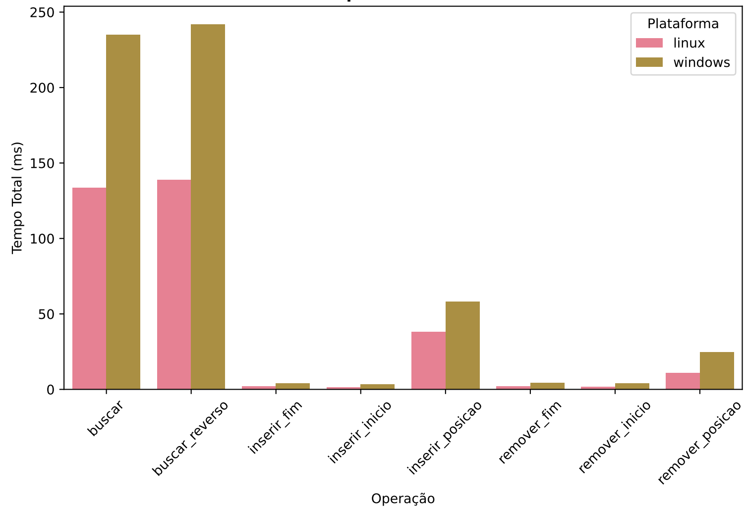
Lista Duplamente Encadeada Circular
