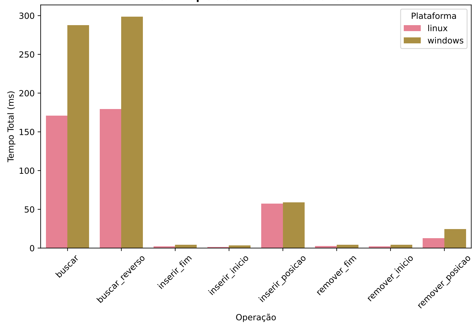
Lista Duplamente Encadeada Circular
