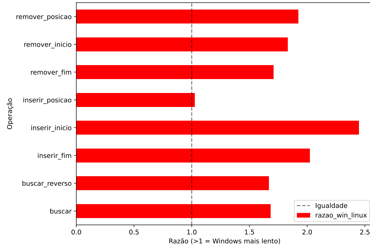
Lista Duplamente Encadeada Circular (Razão Windows/Linux)
