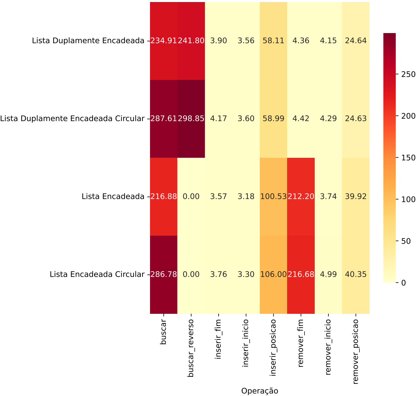
Windows - Tempo Total (ms)
