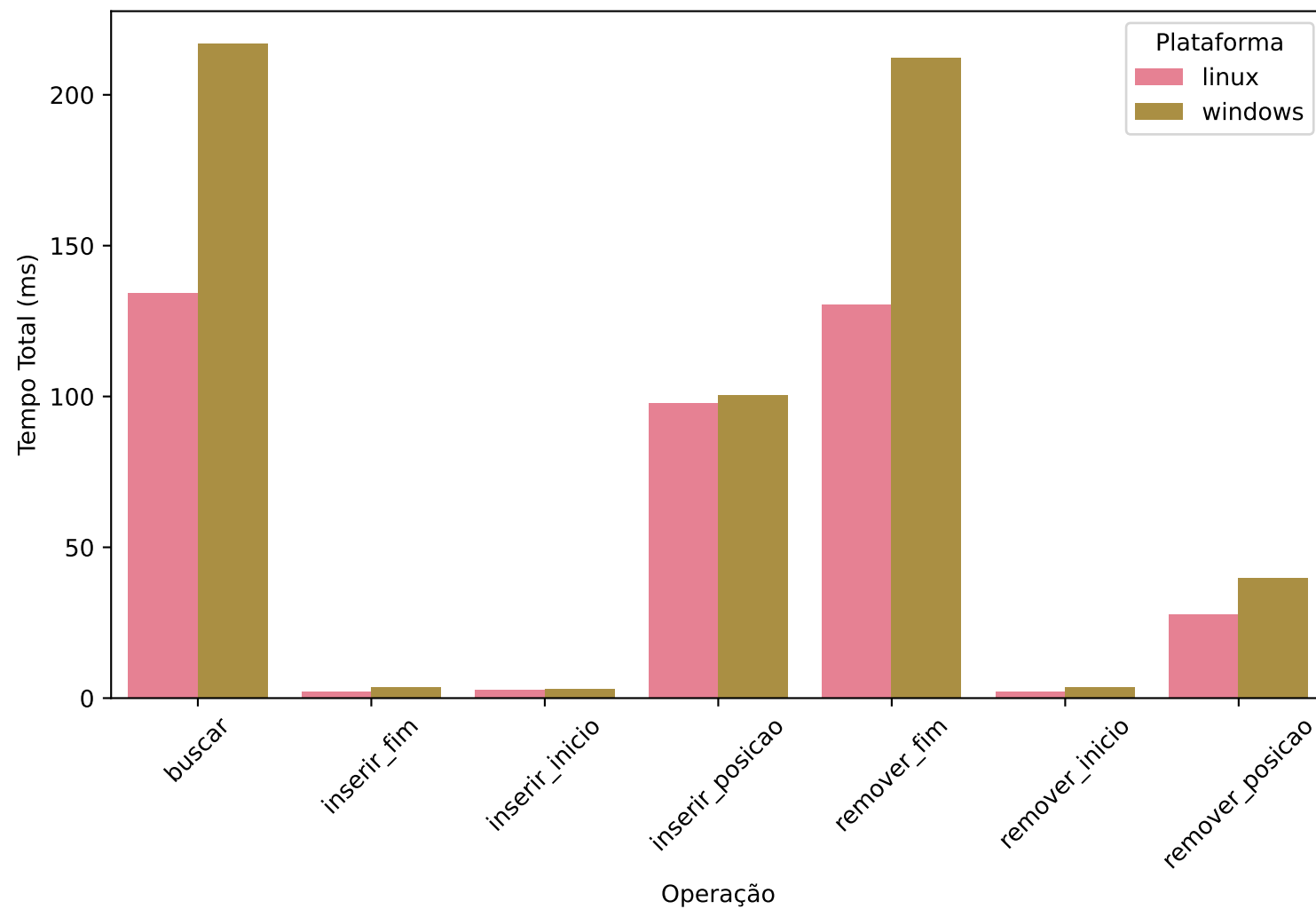
Lista Encadeada Circular
