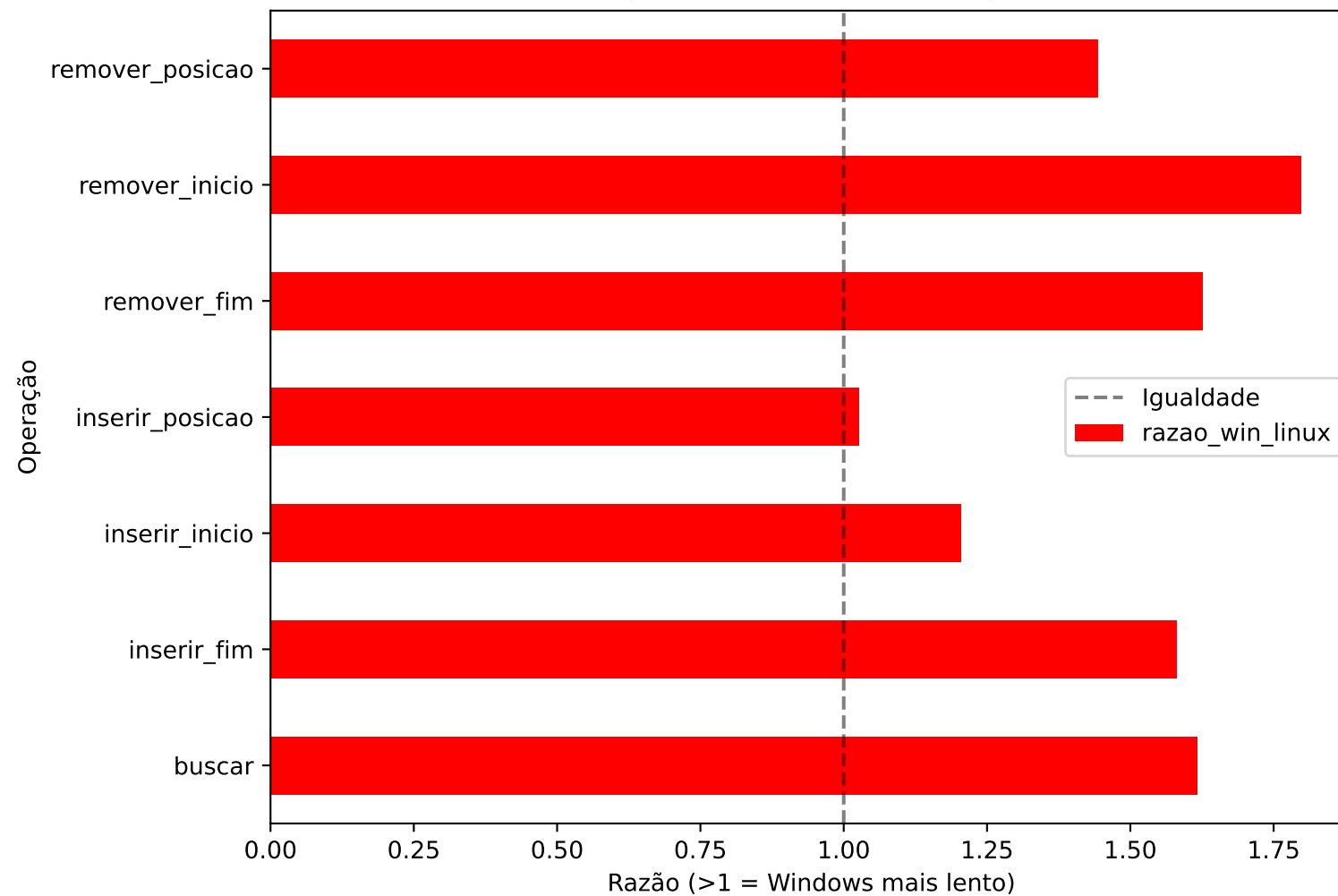
Lista Encadeada Circular (Razão Windows/Linux)
