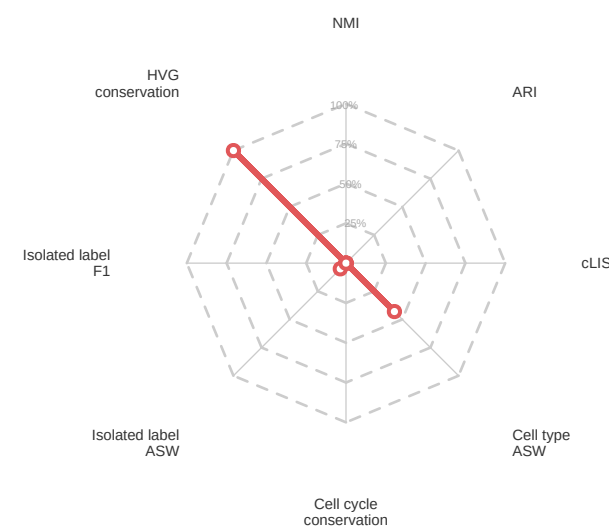
LIGER
