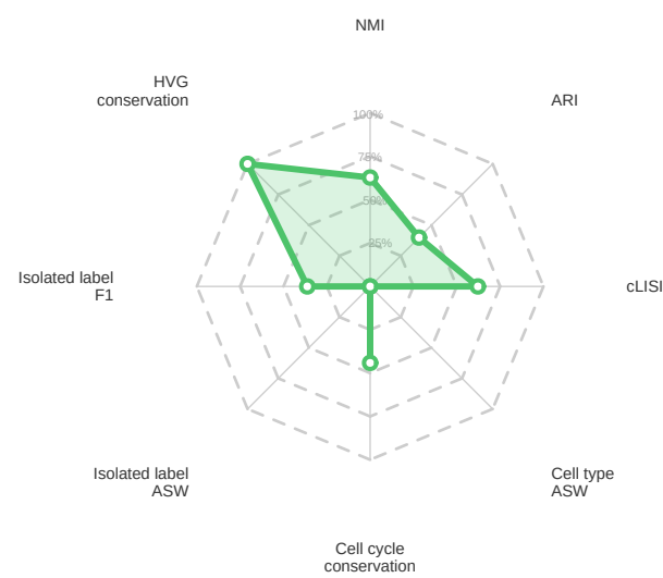
MNN
