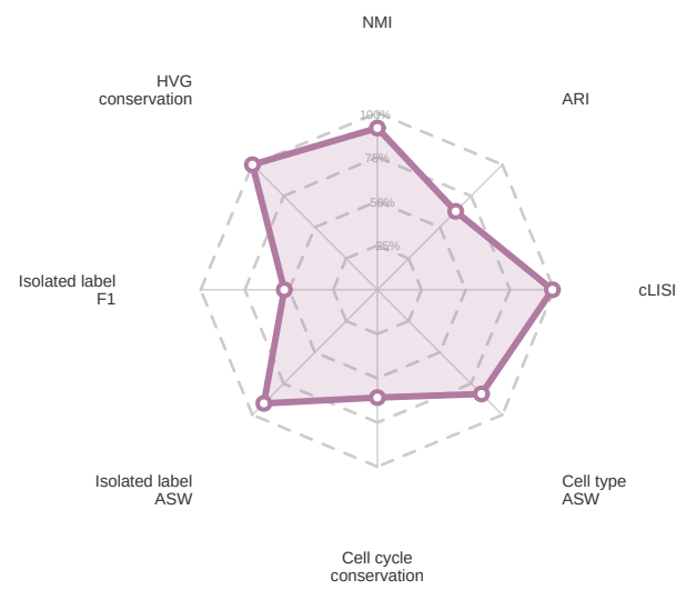
scANVI
