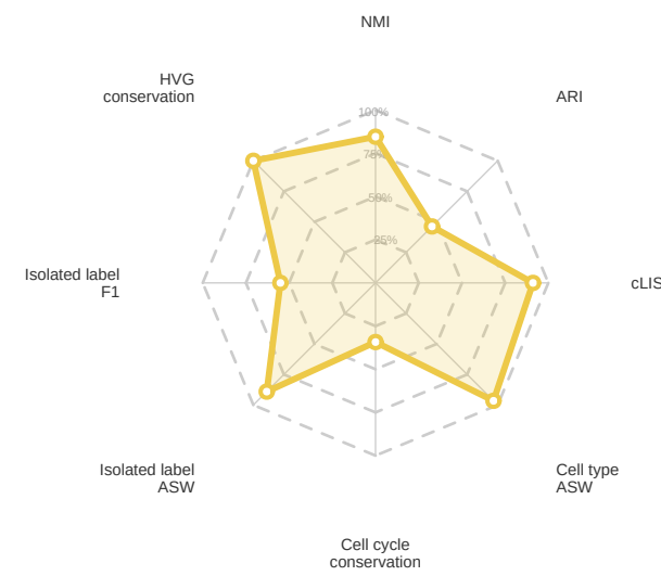
Seurat v5
