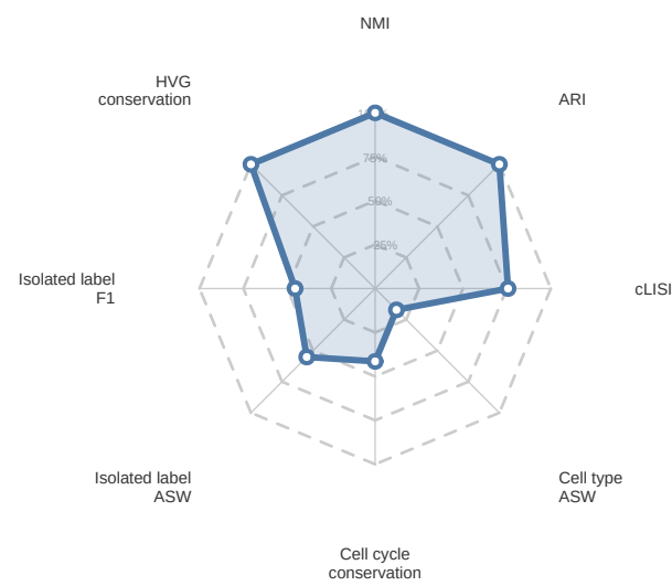
BBKNN
