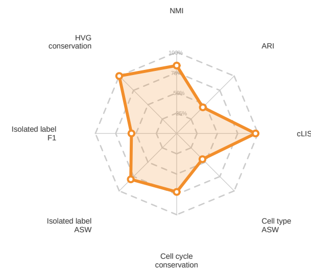
scVI
