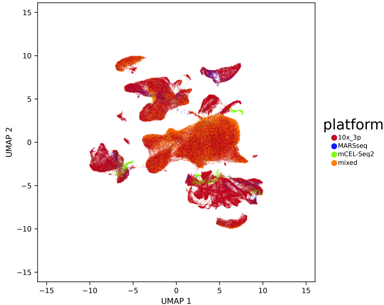
Seurat (RPCA) — seurat_full_hvg_seed0 — platform
