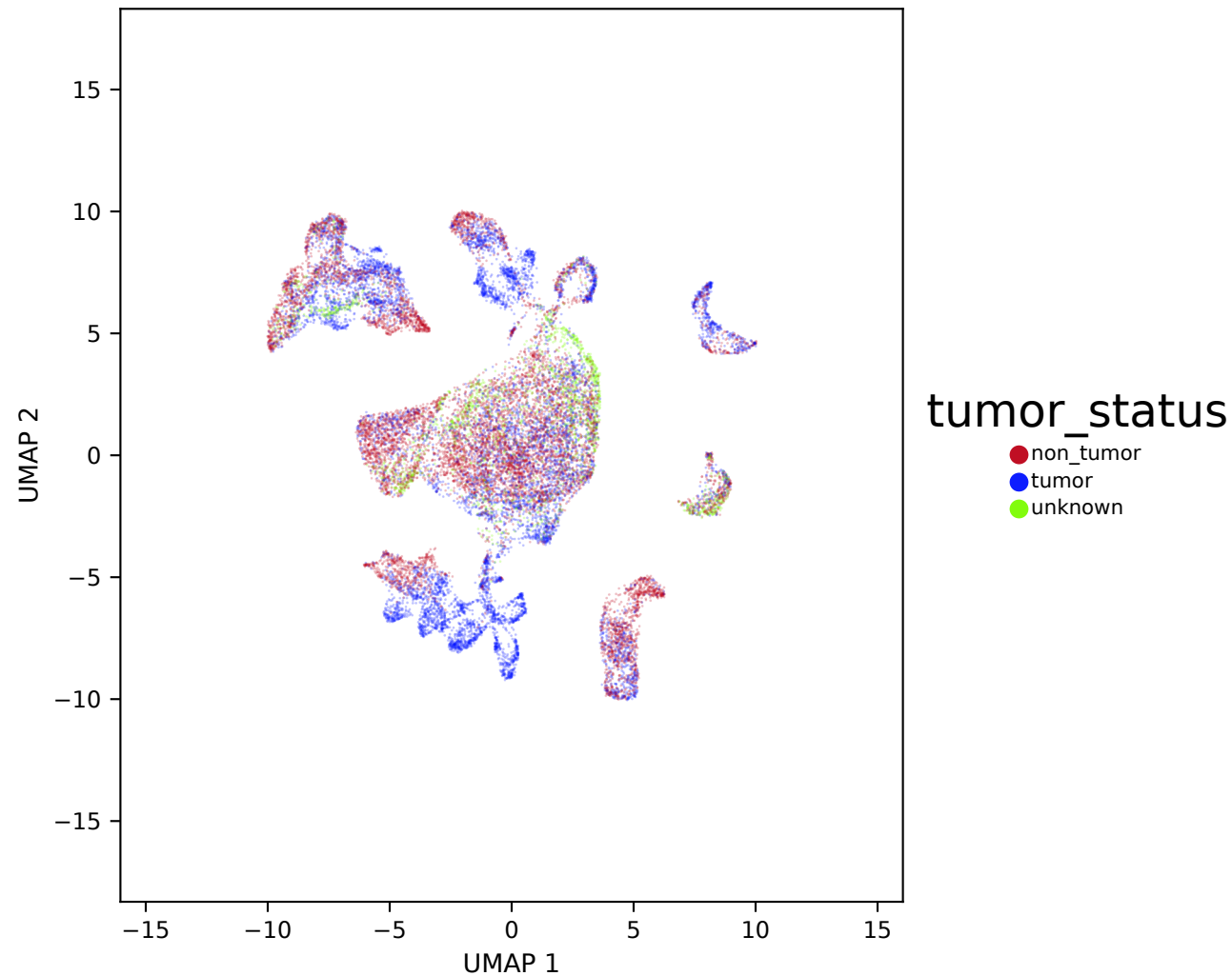
Seurat (RPCA) — seurat_smoke_rpca — tumor status
