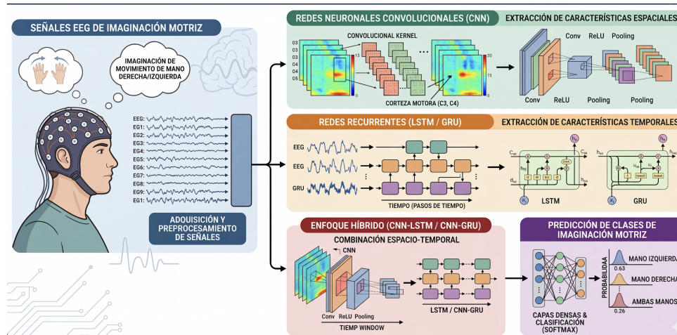
FIGURA 2.2. Estructura general de los modelos y su aplicación en la clasificación de tareas de imaginación motriz.
