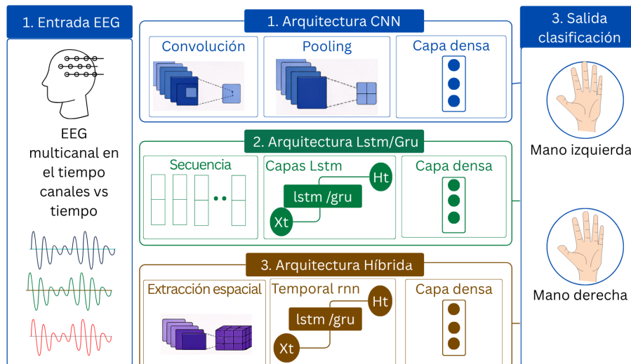
FIGURA 2.2. Estructura general de los modelos y su aplicación en la clasificación de tareas de imaginación motriz 1 .
