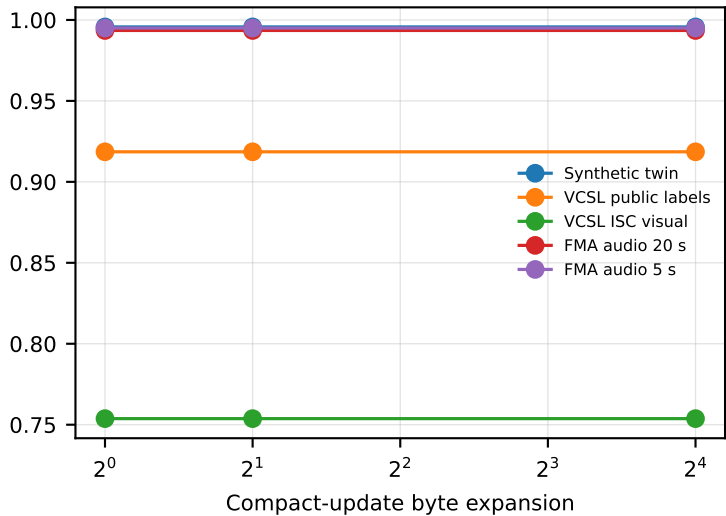
PR-AUC
