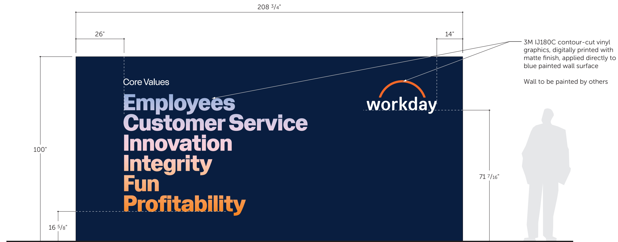
WALL GRAPHIC Scale: 3/8" = 1' - 0"
