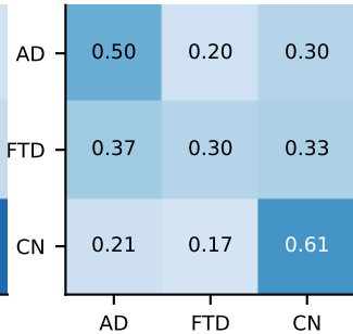
P4×spatial F1=0.46
