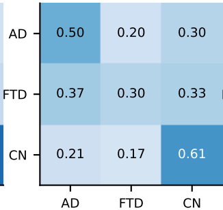
P4×spatial F1=0.46
