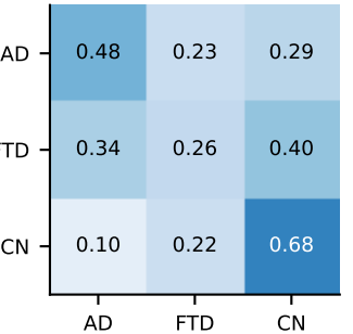
P7×spatial F1=0.45
