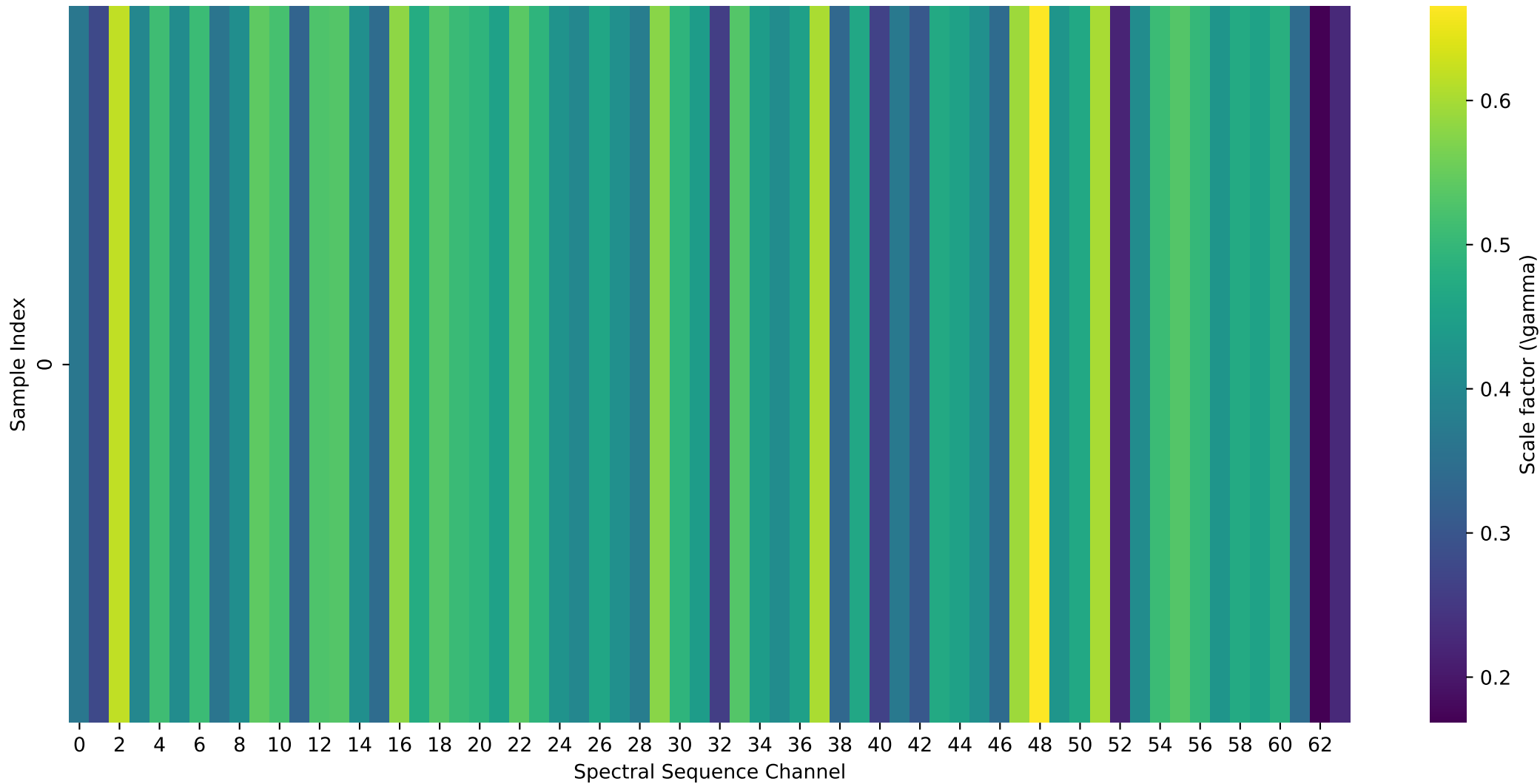
PaviaU BiGRU Scale ( \gamma )
