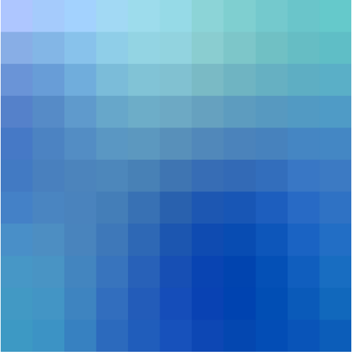
True: Bitumen
