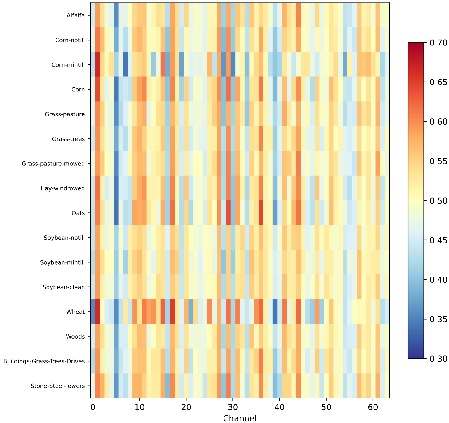
Mean \gamma (Scale)
