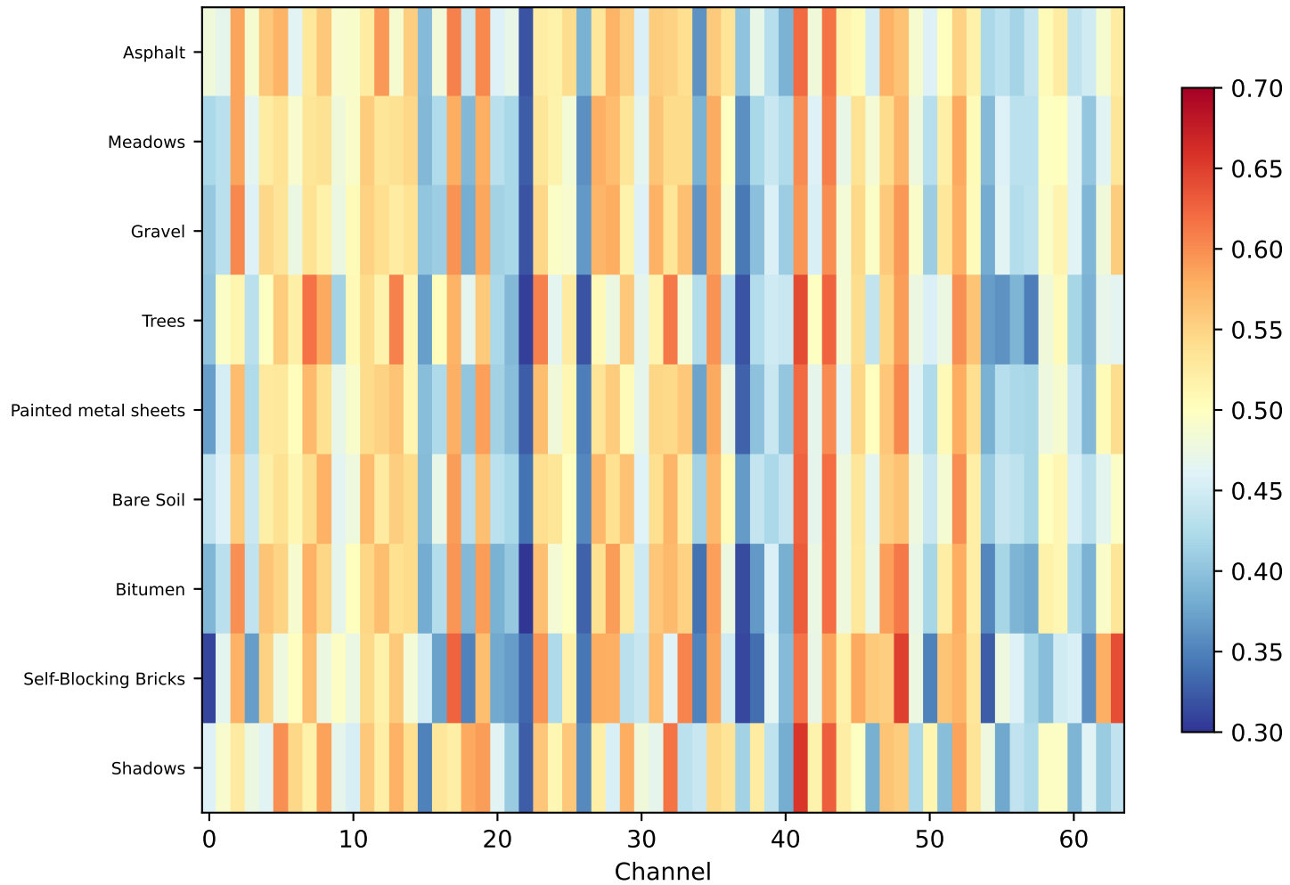
Mean \gamma (Scale)
