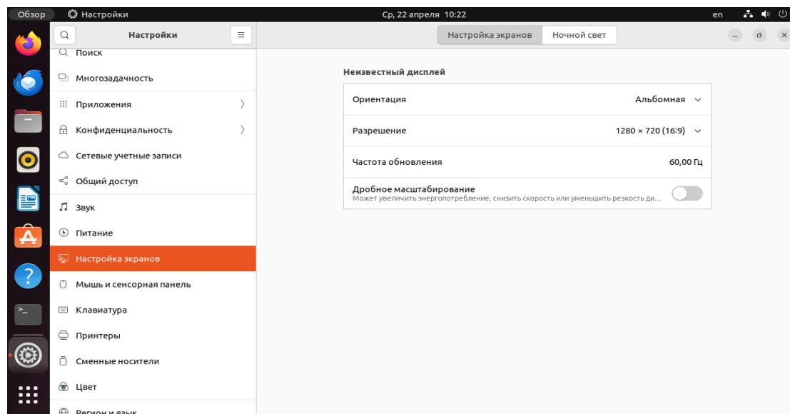
Ubuntu 22.04.4 LTS
