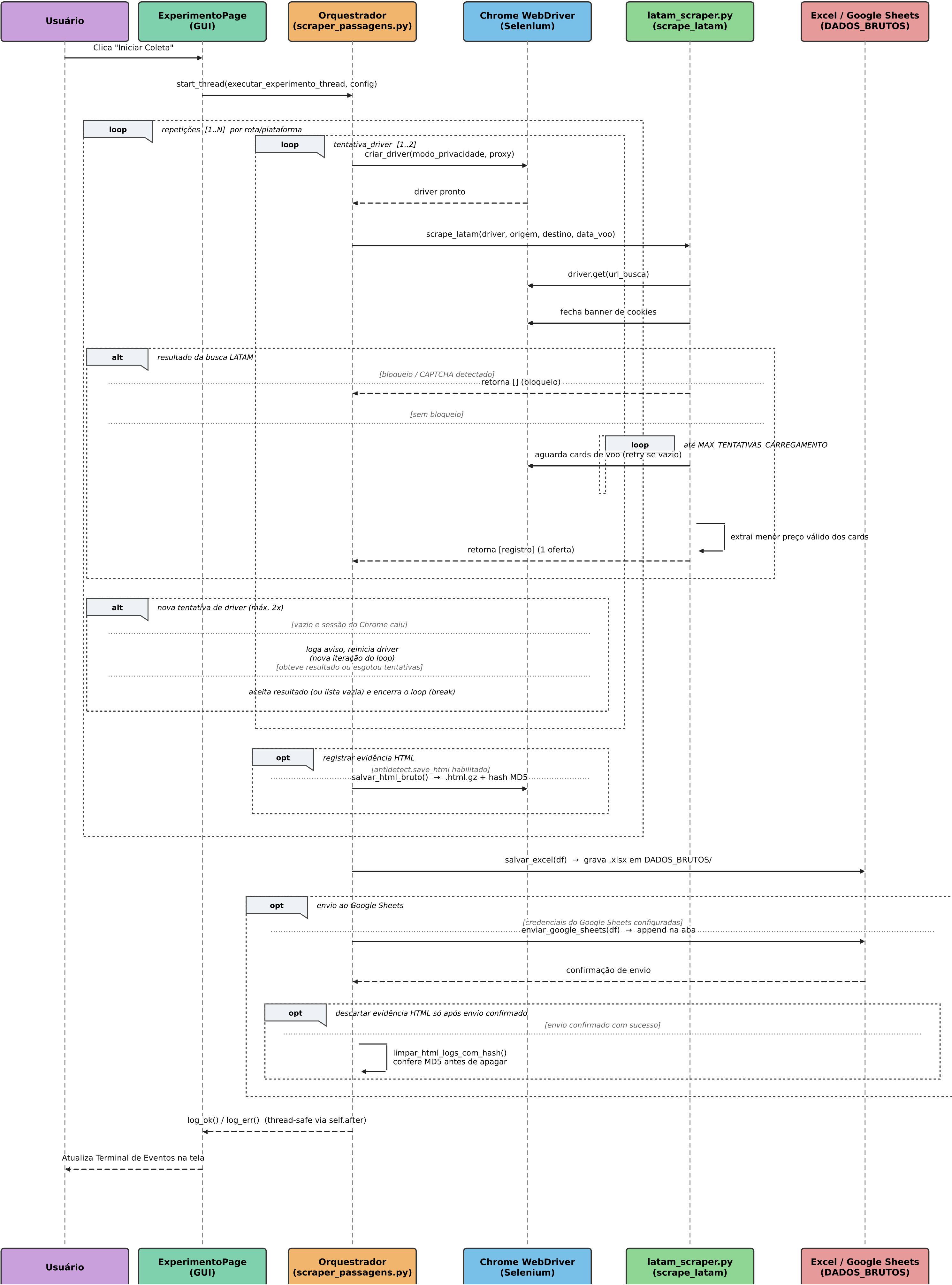
Diagrama de Sequência — Pipeline de Coleta e Persistência (AirPrice)
