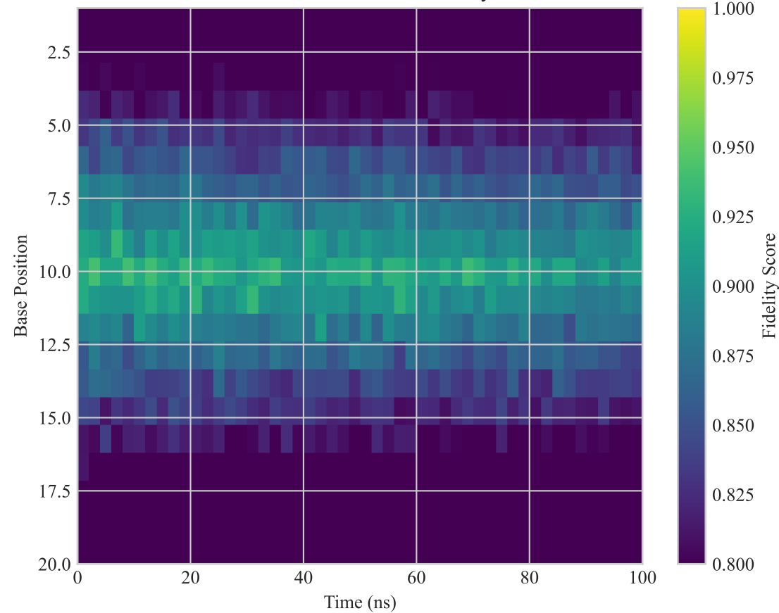
A. Cas12b Base-Pair Fidelity
