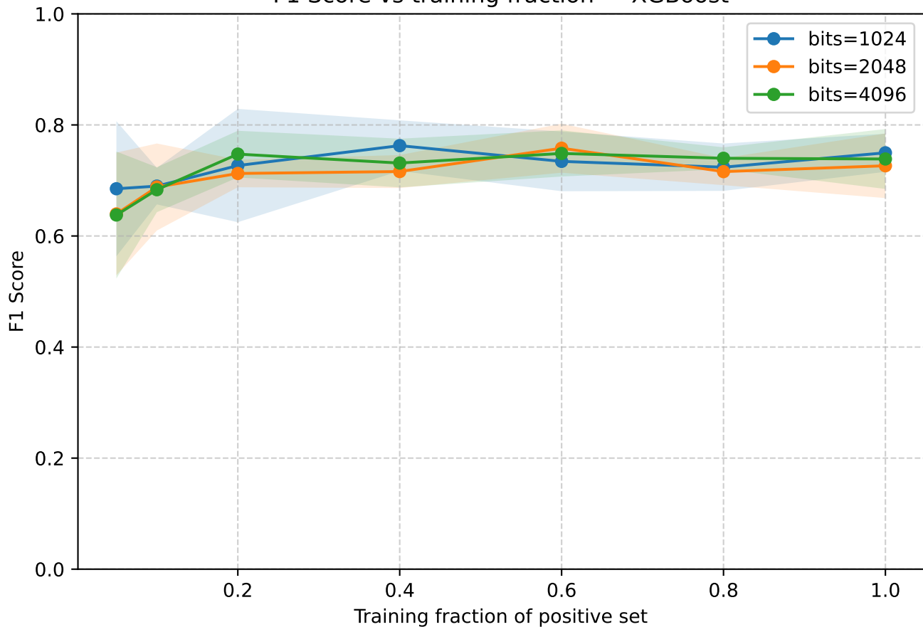
F1 Score vs training fraction — XGBoost
