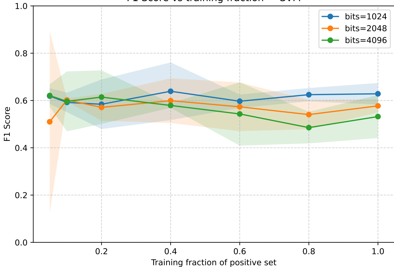
F1 Score vs training fraction — SVM
