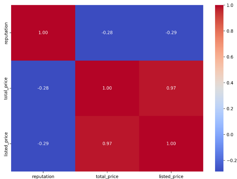
Рисунок 14 - Корреляционная матрица
