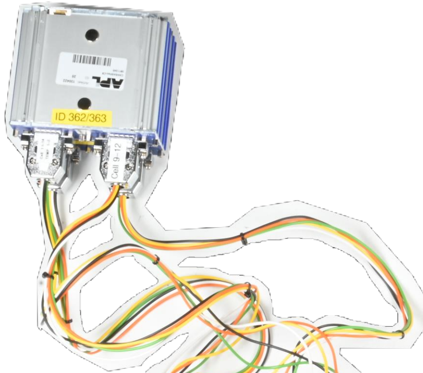
CANSAS-Module
