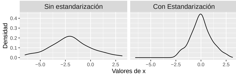
Figura 4.1: Estandarización de una variable con distribución Normal
