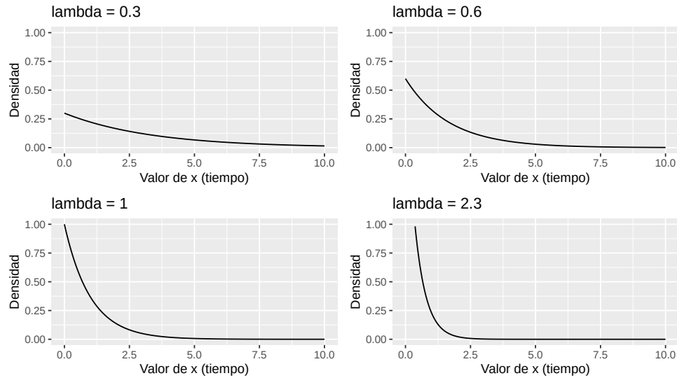
Figura 3.11: Simulación de la distribución Exponencial
