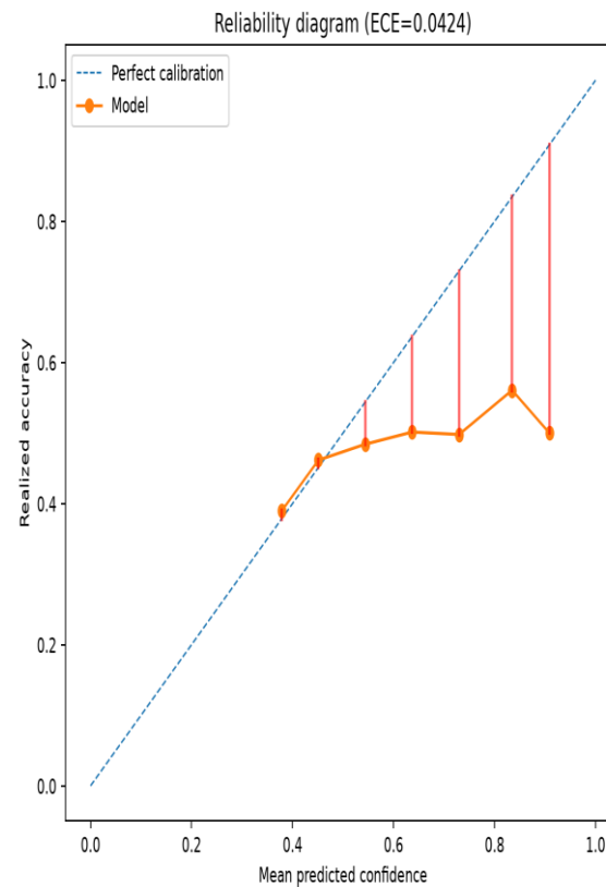
calibration.png
