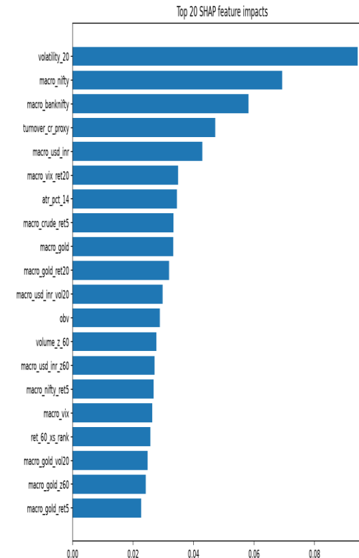
shap_summary.png
