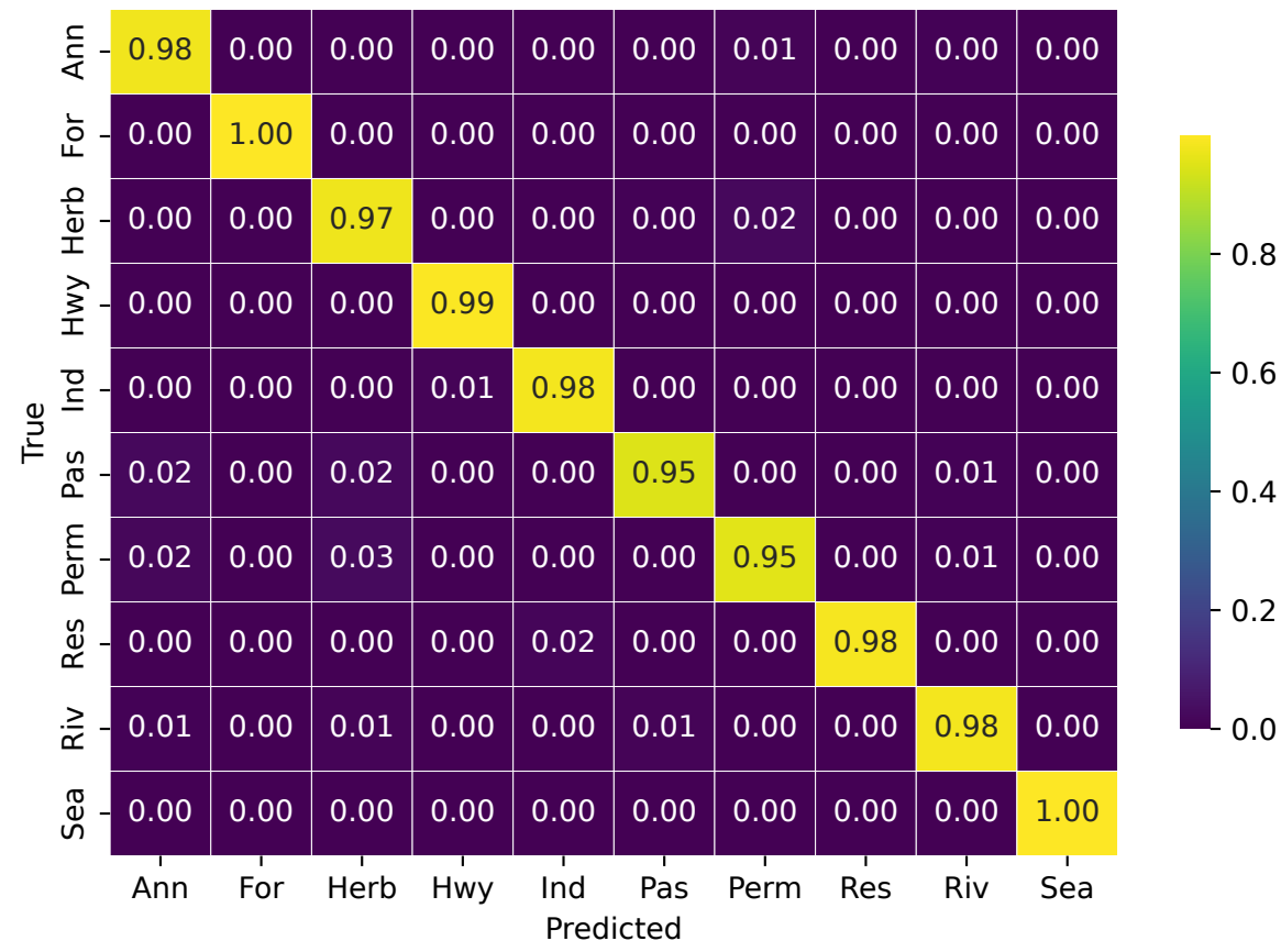
EXP-C — Uniform 8q VQC (OA=0.9761)
