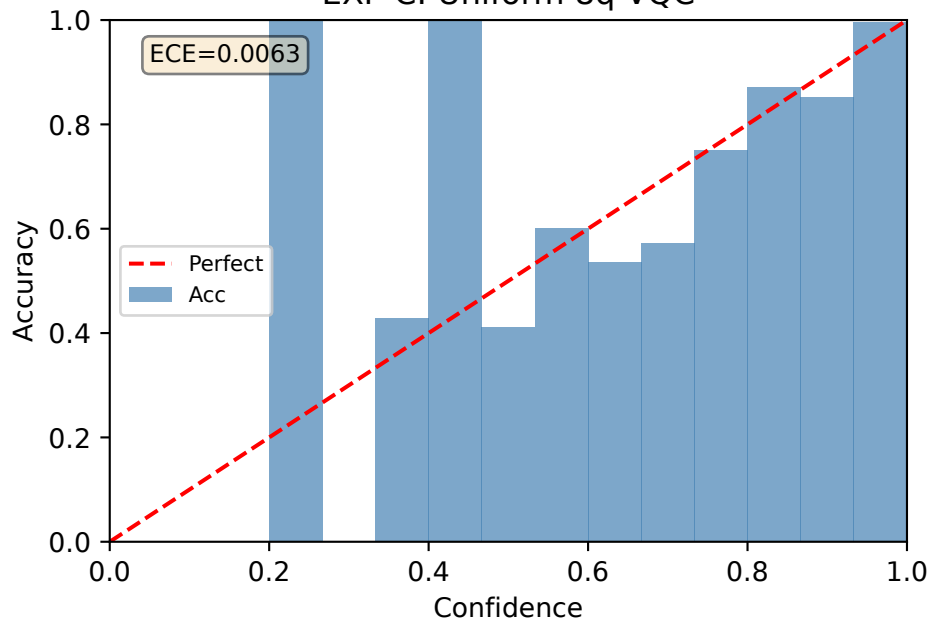
EXP-C: Uniform 8q VQC
