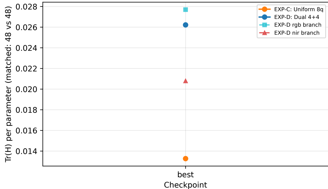
Tr(H) per parameter (matched: 48 vs 48)
