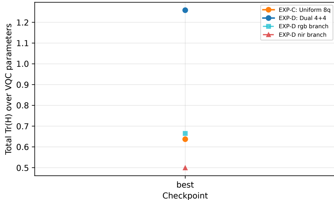
Total Tr(H) over VQC parameters
