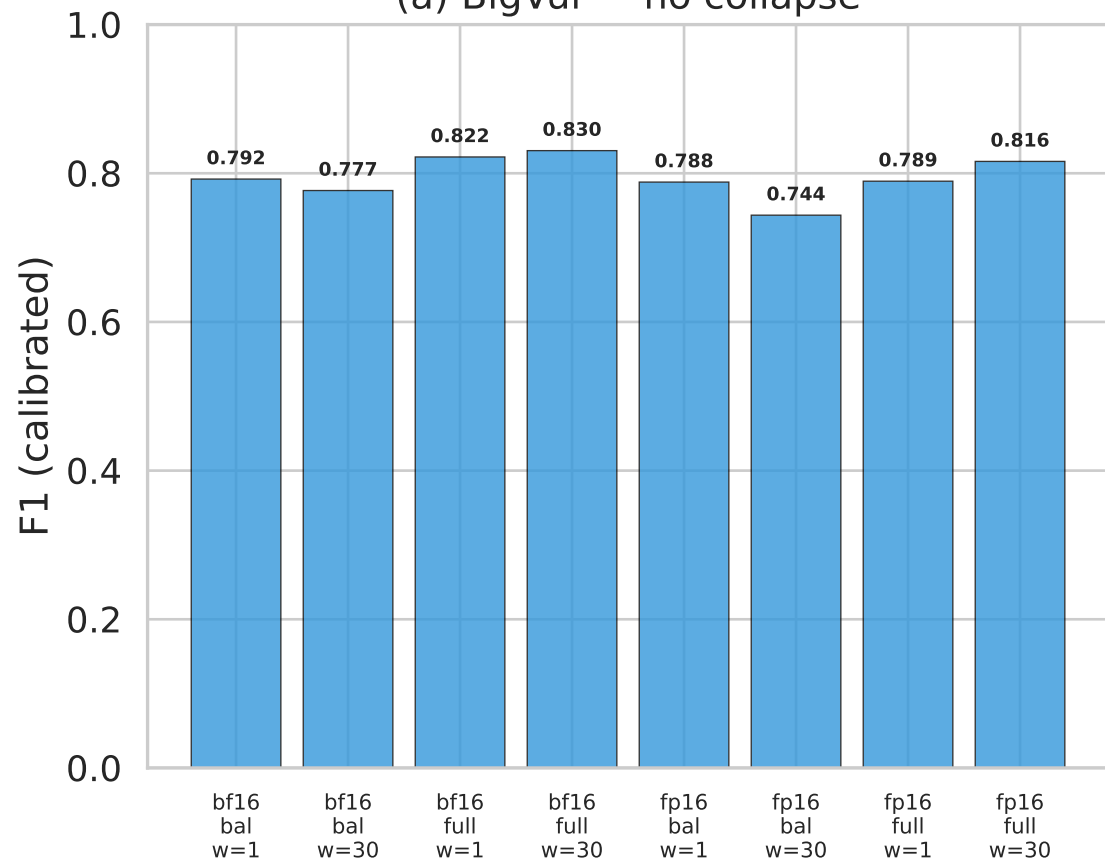
(a) BigVul — no collapse
