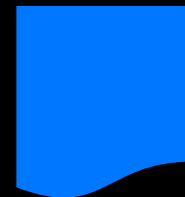
Плохой шаблон
