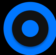
Выдумка
