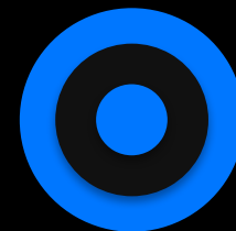
Перегрузка
