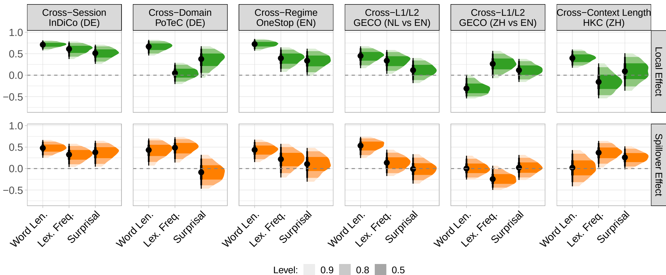
Posterior Correlation Coefficient
