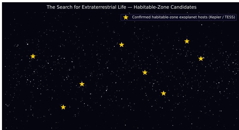
איור 1: חיפוש חיים חוץ-ארציים: מועמדי אזור מגורים בגלקסיה (Kepler / TESS)
