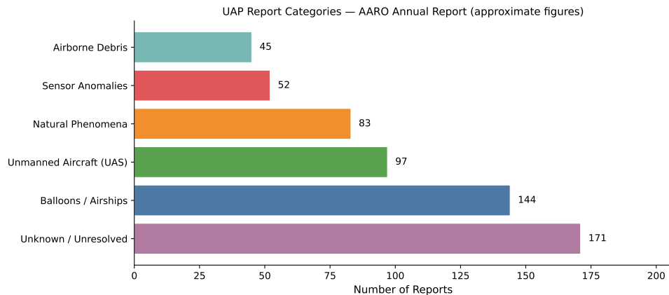
איור 2: התפלגות קטגוריות UAP לפי דיווחי AARO (נתונים משוערים)
