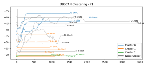
Figura 7. Clusters formados con el metodo DBSCAN utilizando todos los features seleccionados.
