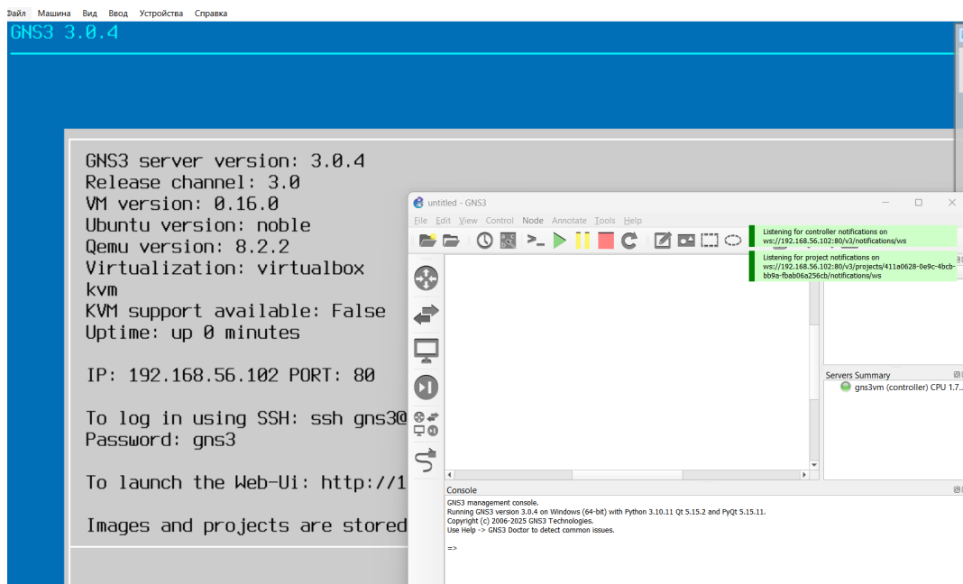
Рис. 2.16: Настроенная gns3
