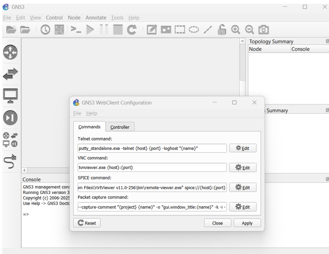
Рис. 2.13: Приложение gns3
