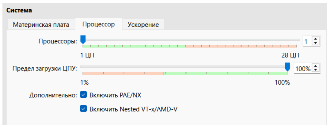
Рис. 2.10: Команда выполнена
