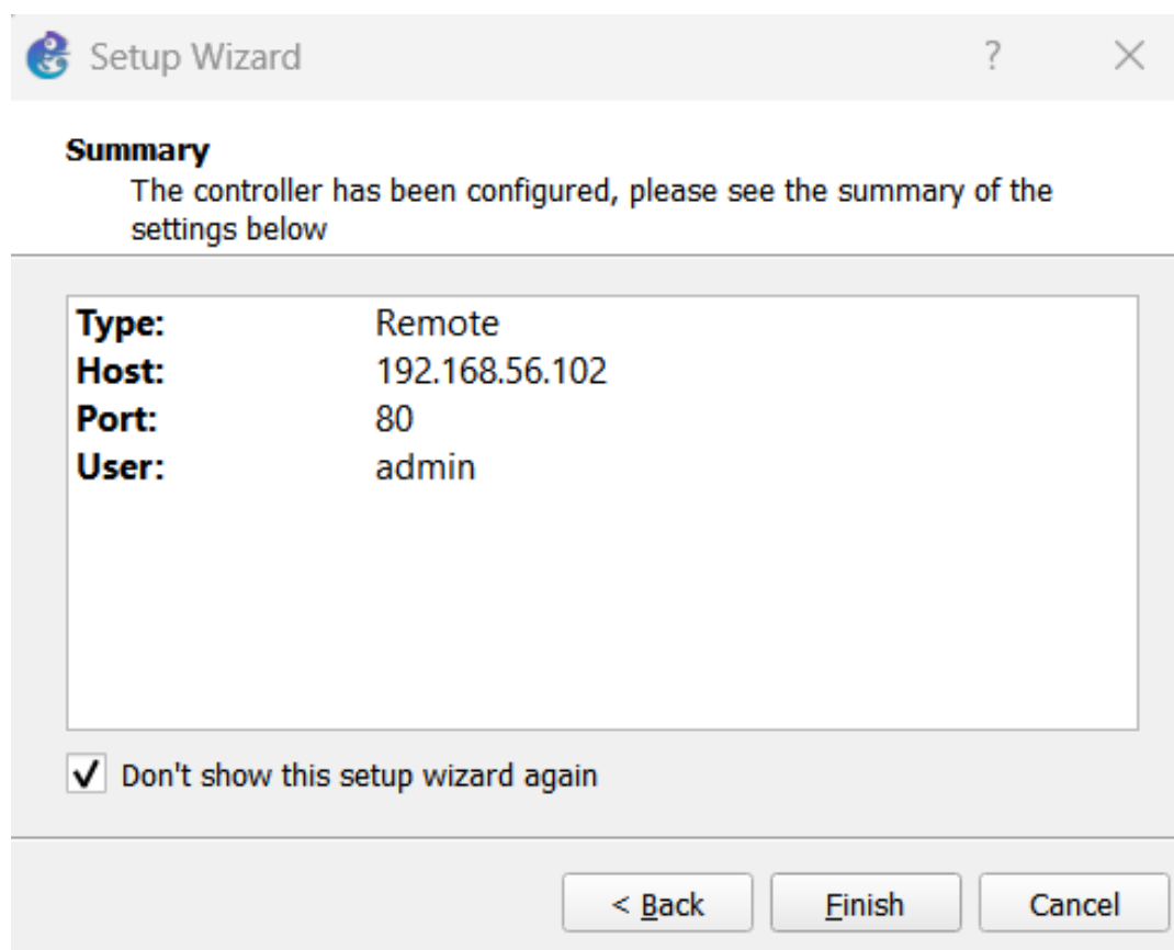
Рис. 2.15: Настройка
