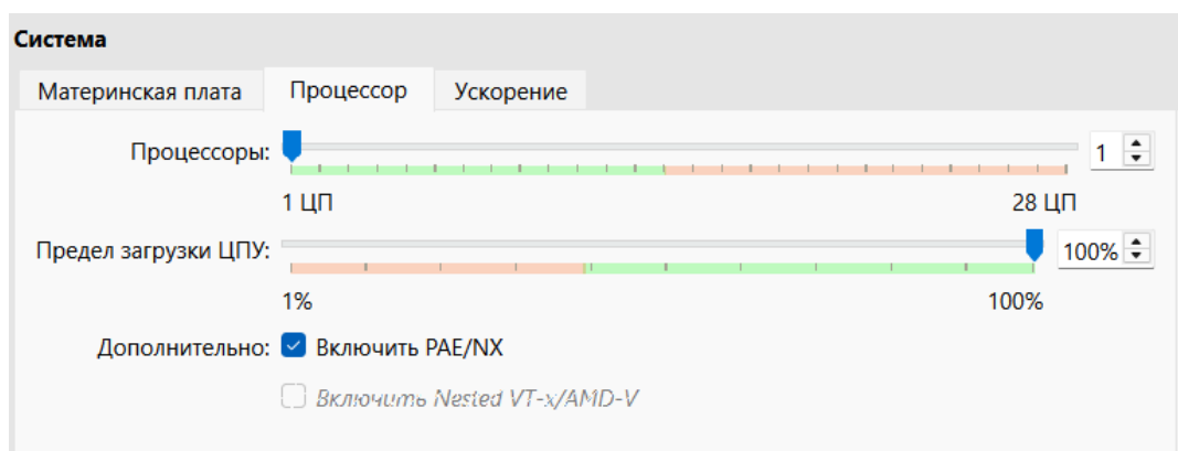
Рис. 2.8: Окно настройки
