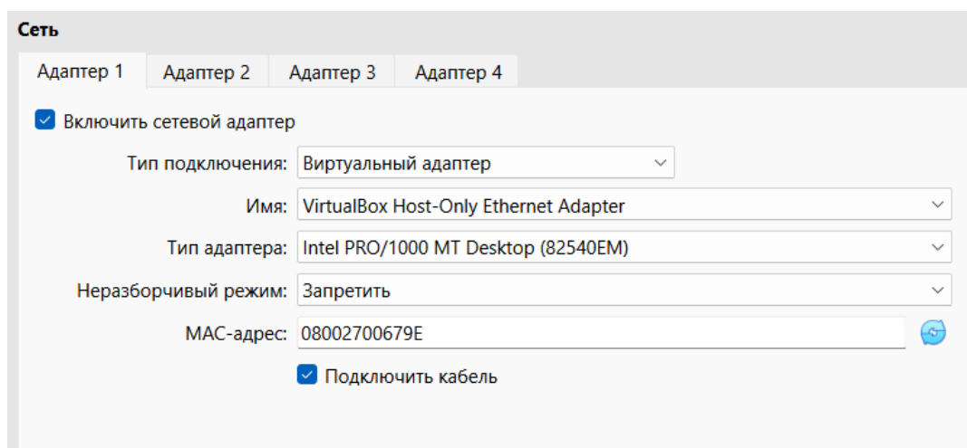
Рис. 2.11: Адаптер 1
