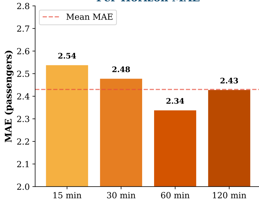
Per-Horizon MAE
