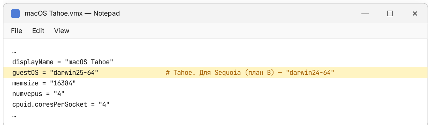
Рис. 17. Ключевые строки файла .vmx. guestOS должен соответствовать версии macOS в образе.
