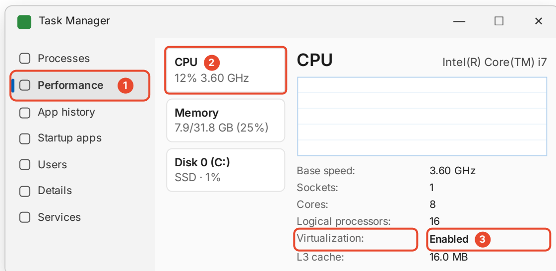
Рис. 1. Диспетчер задач → Производительность → ЦП. Строка «Virtualization / Виртуализация» должна показывать «Enabled / Включено».
