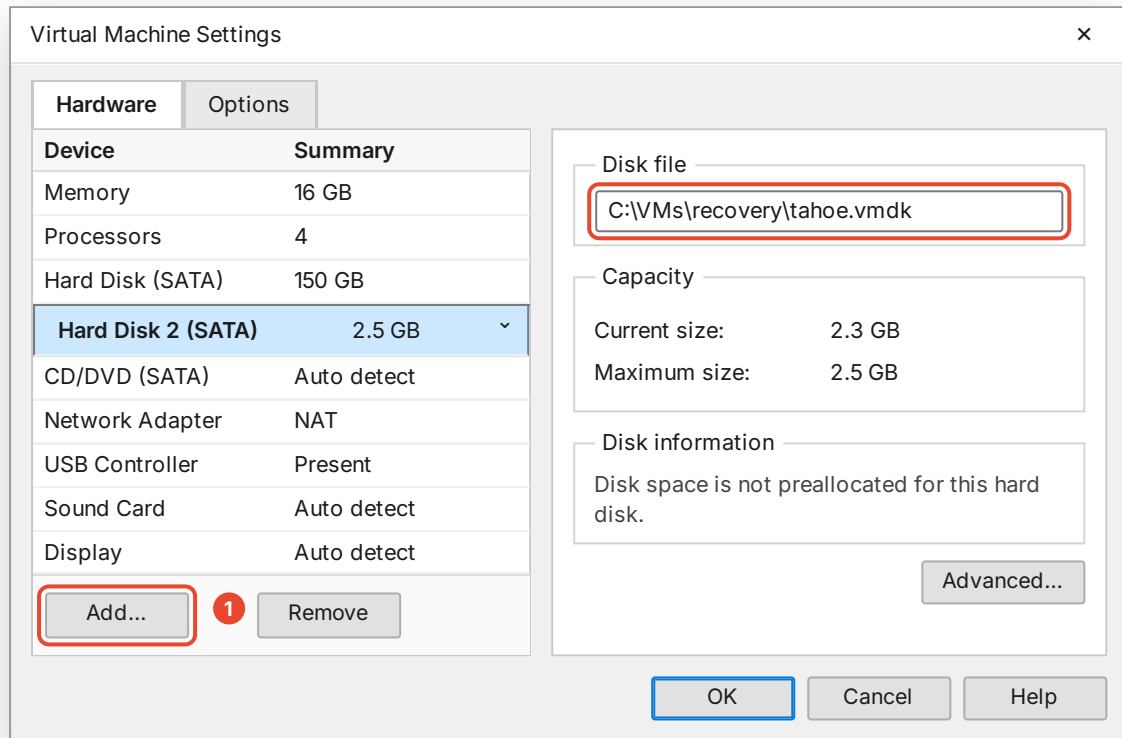
Рис. 16. Итоговые настройки: основной диск на 150 ГБ и второй диск — образ восстановления tahoe.vmdk.
