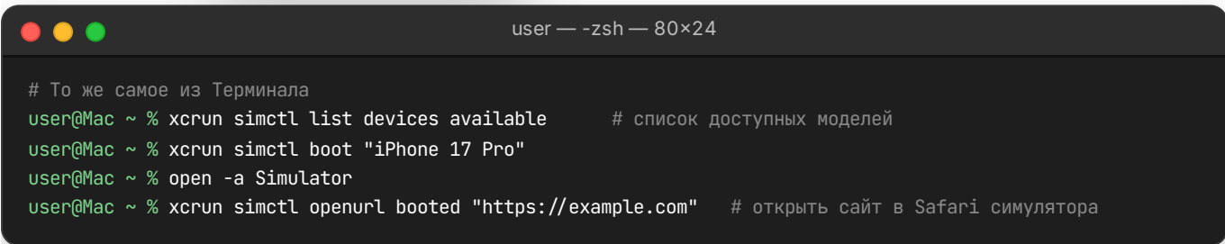
Рис. 26. Управление симулятором из Терминала.
