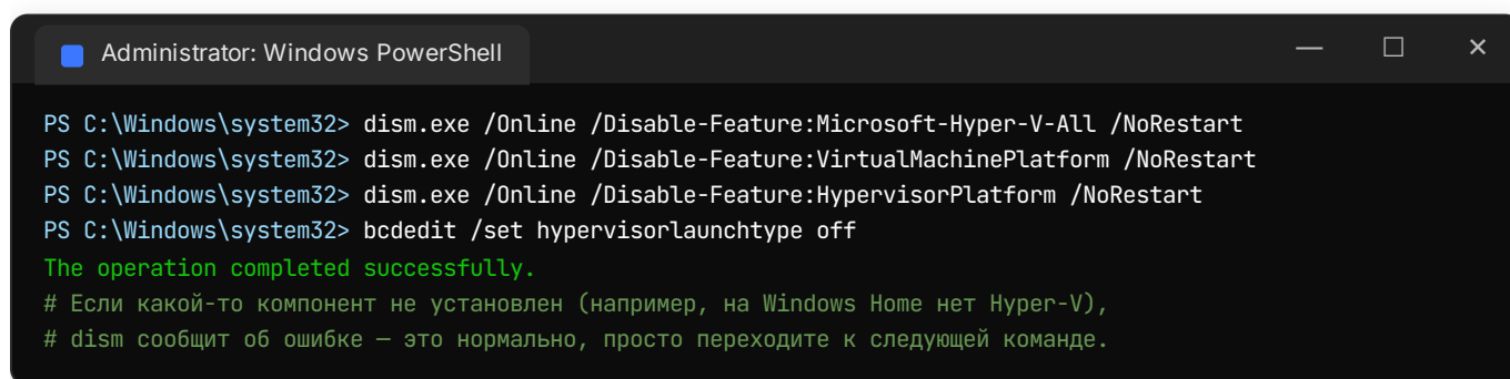
Рис. 3. Команды для отключения Hyper-V, платформы виртуальных машин и гипервизора Windows.
