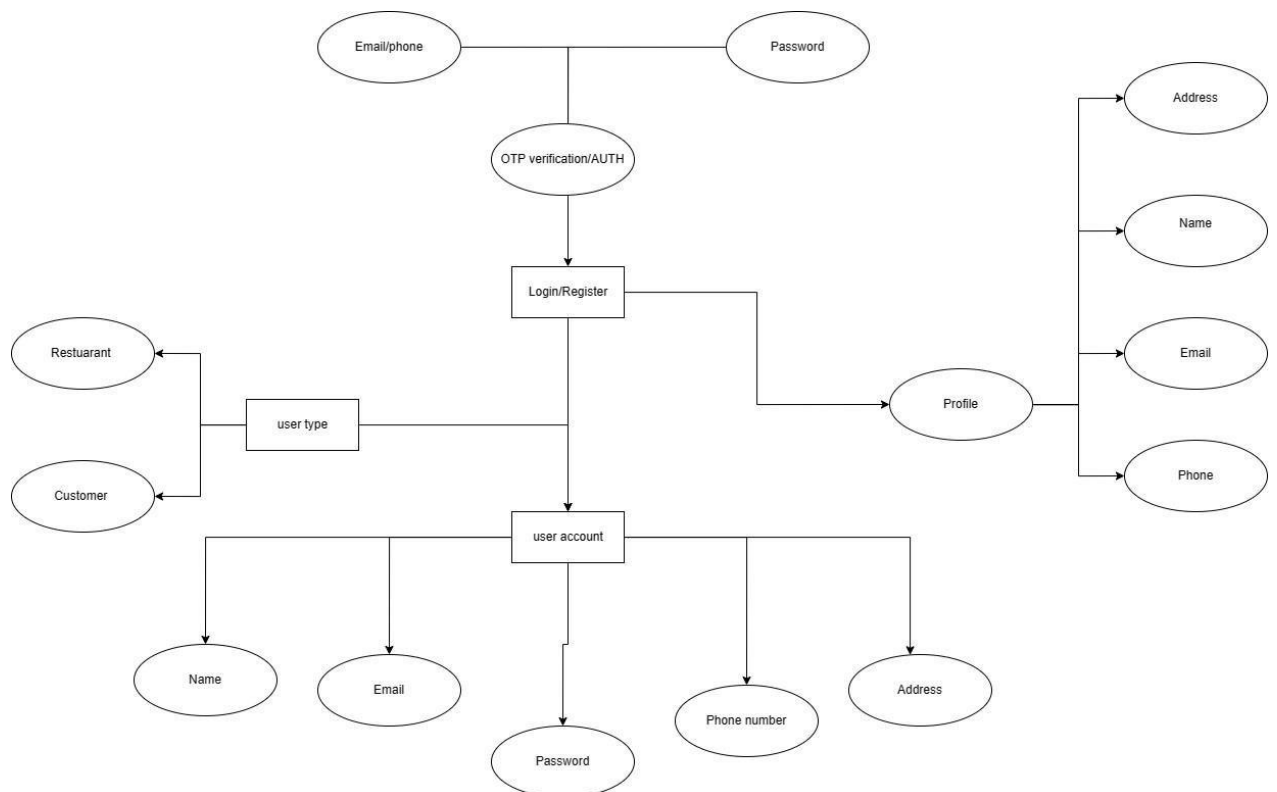
Figure 5 ERD UM
