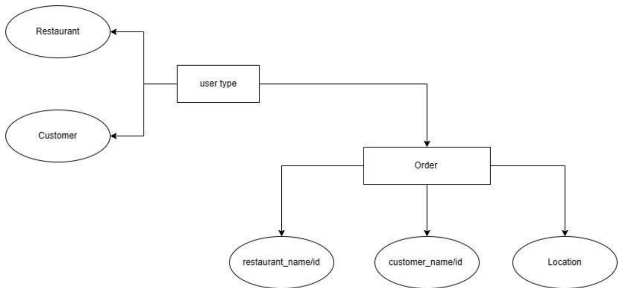
Figure 15 ERD OM
