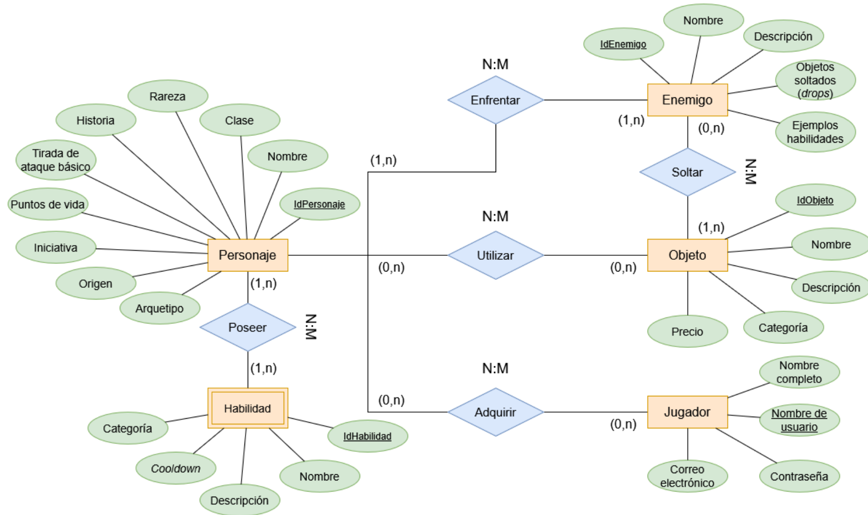
Figura 14: Representación del modelo entidad-relación
