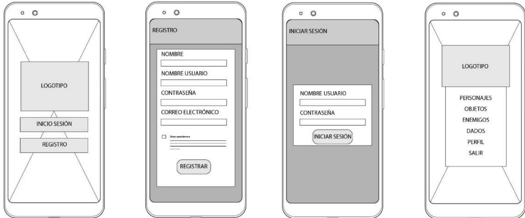
Figura 38: Wireframes de las pantallas: Acceso, Registro, Inicio de sesión e Inicio
