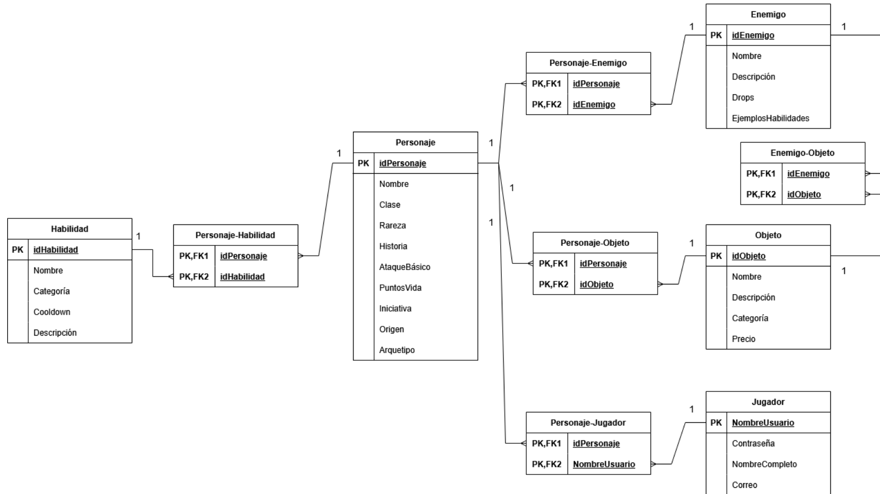
Figura 15: Representación del modelo relacional
