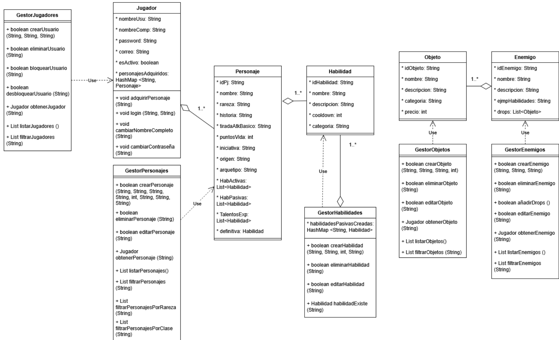
Figura 37: Diagrama de clases
