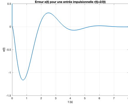
(a) e(t) pour r_1(t) = 2\delta(t) .
