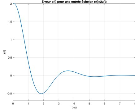
(a) e(t) pour r_2(t) = 2H(t) .
