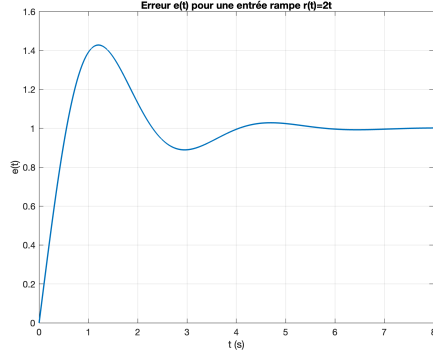
(a) e(t) pour r_3(t) = 2t .
