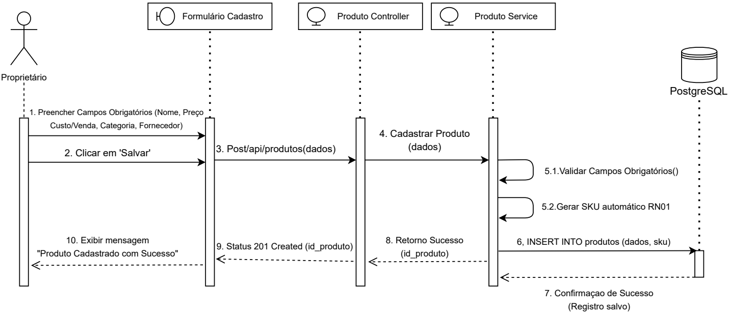
Diagrama de Sequência: Cadastro de Produto
