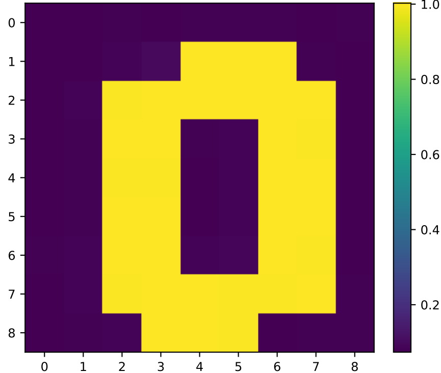
razón \rho = mediana / iluminación
