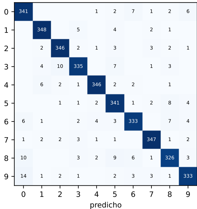
matriz de confusión (validación)
