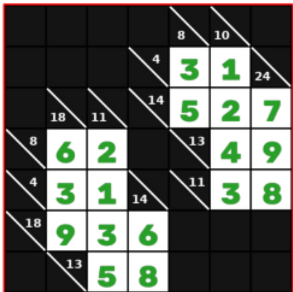
✓ 06_photo_dim
