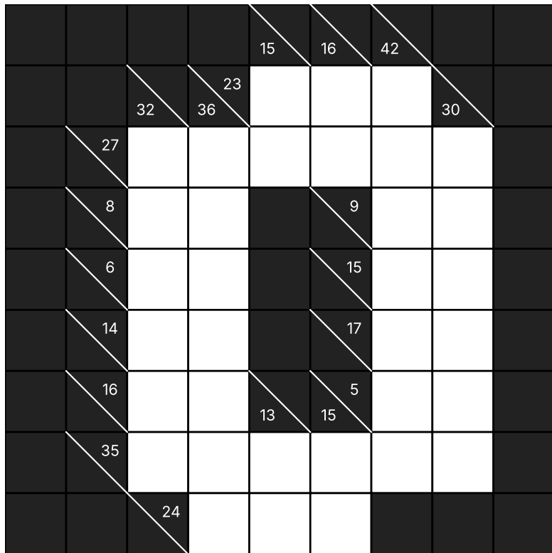
puzzle extraído
