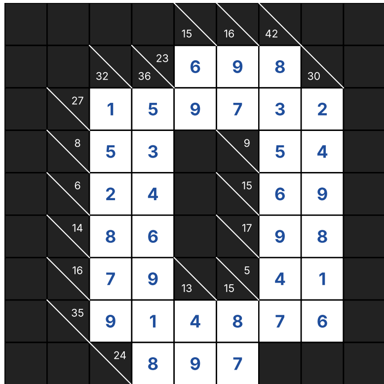
solución CP
