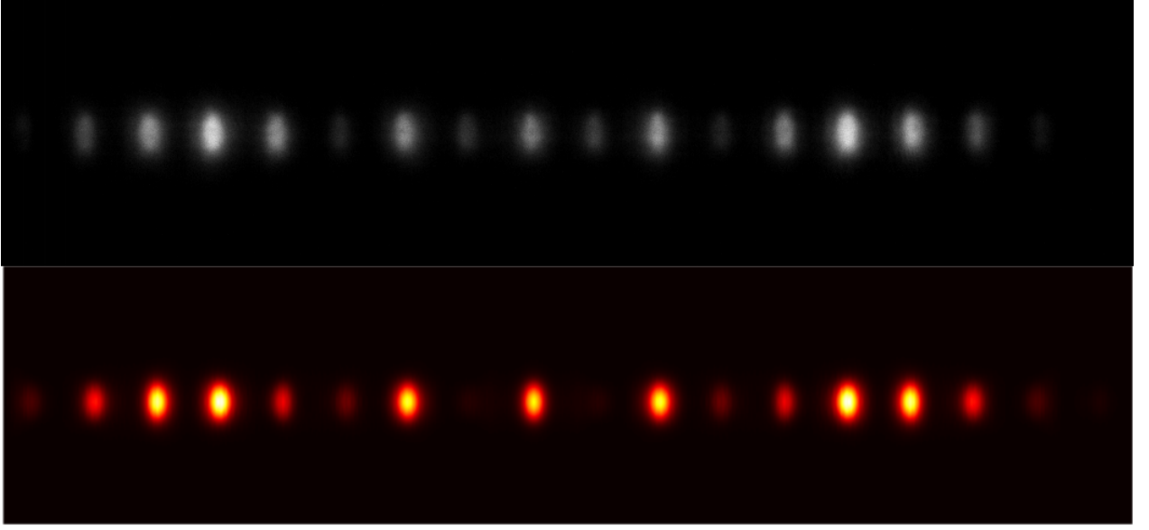
Figura 3.2: Excitación del sitio central de una red unidimensional. Arriba: Medición experimental a \lambda = 730 nm. Abajo: Simulación numérica realizada con BPM.
