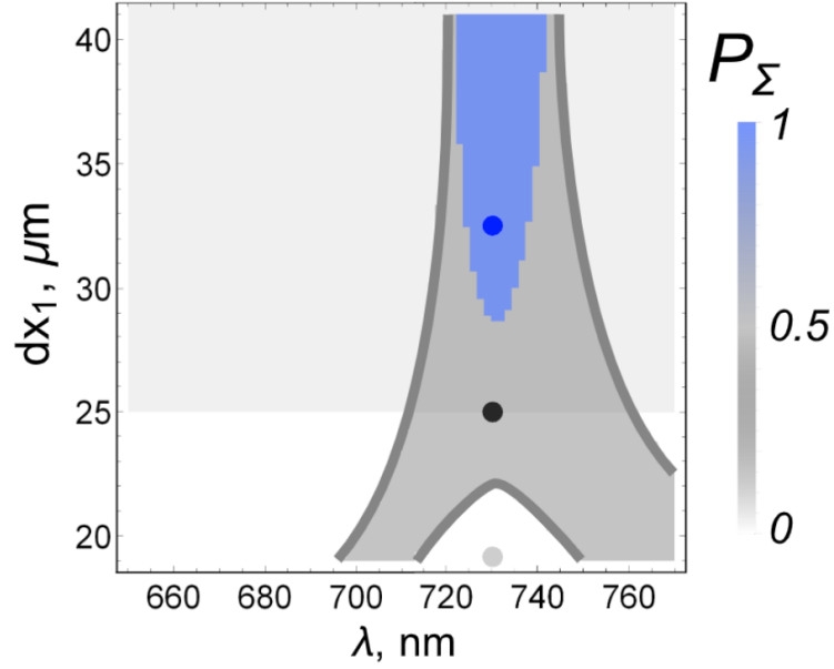
Figura 7.5: Diagrama de fases topológicas.
