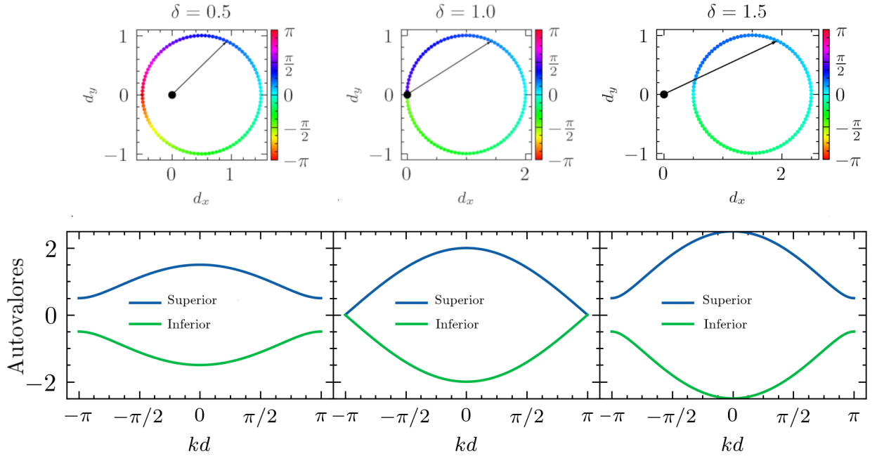
Figura 2.6: Topología de la red SSH. Arriba: Vectores \mathbf{d}(k) y su fase. Para \delta < 1 ( \delta > 1 ), (no) se encierra el origen. Abajo: Bandas en función del cuasimomento k en la primera zona de Brillouin para \delta < 1 , \delta = 1 y \delta > 1 . Se fija t' = 1 y se varía \delta' para un número N = 100 de celdas unitarias.
