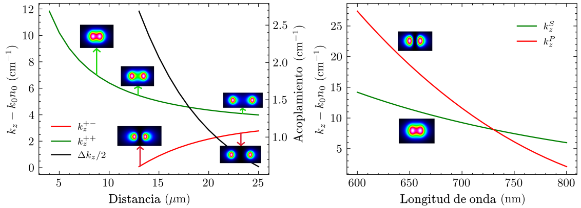
Figura 7.2: Izquierda: Constantes de propagación y acoplamientos en función de la distancia para modos fundamentales, calculados mediante EME. Derecha: Constantes de propagación de modos S y P en función de la longitud de onda.
