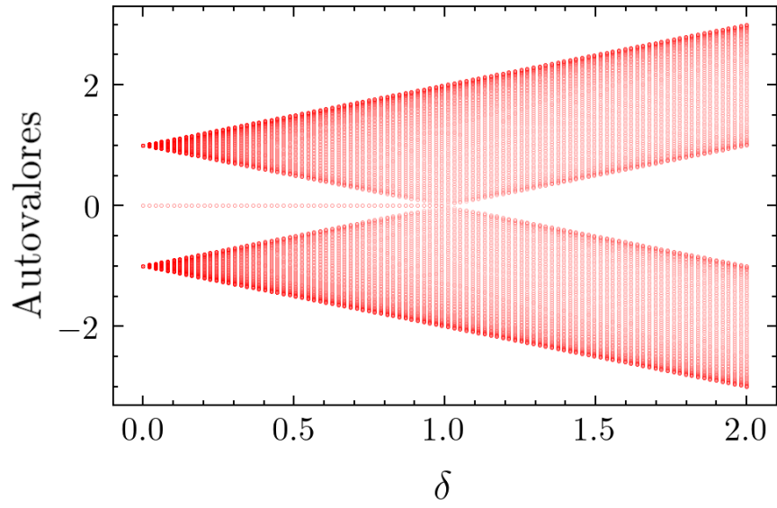
Figura 2.7: Espectro de la red SSH finita. Se aprecia la aparición de los estados de borde a energía cero para \delta < 1 . Condiciones de borde abiertas en función del parámetro \delta = t/t' , para t' = 1 fijo y para un número N = 100 de celdas unitarias.
