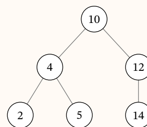
Dopo: 10 sostituisce 8
