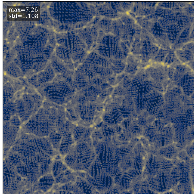
cnn_wst efficient-thunder-86
