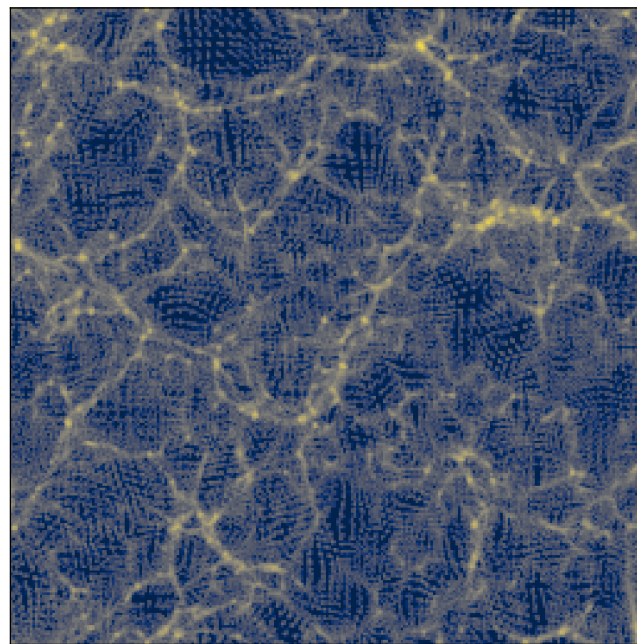
cnn_wst efficient-thunder-86
